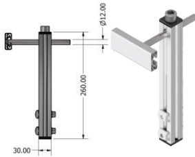
ALUMINIUM HOLDER 30X30 + PROFIL
